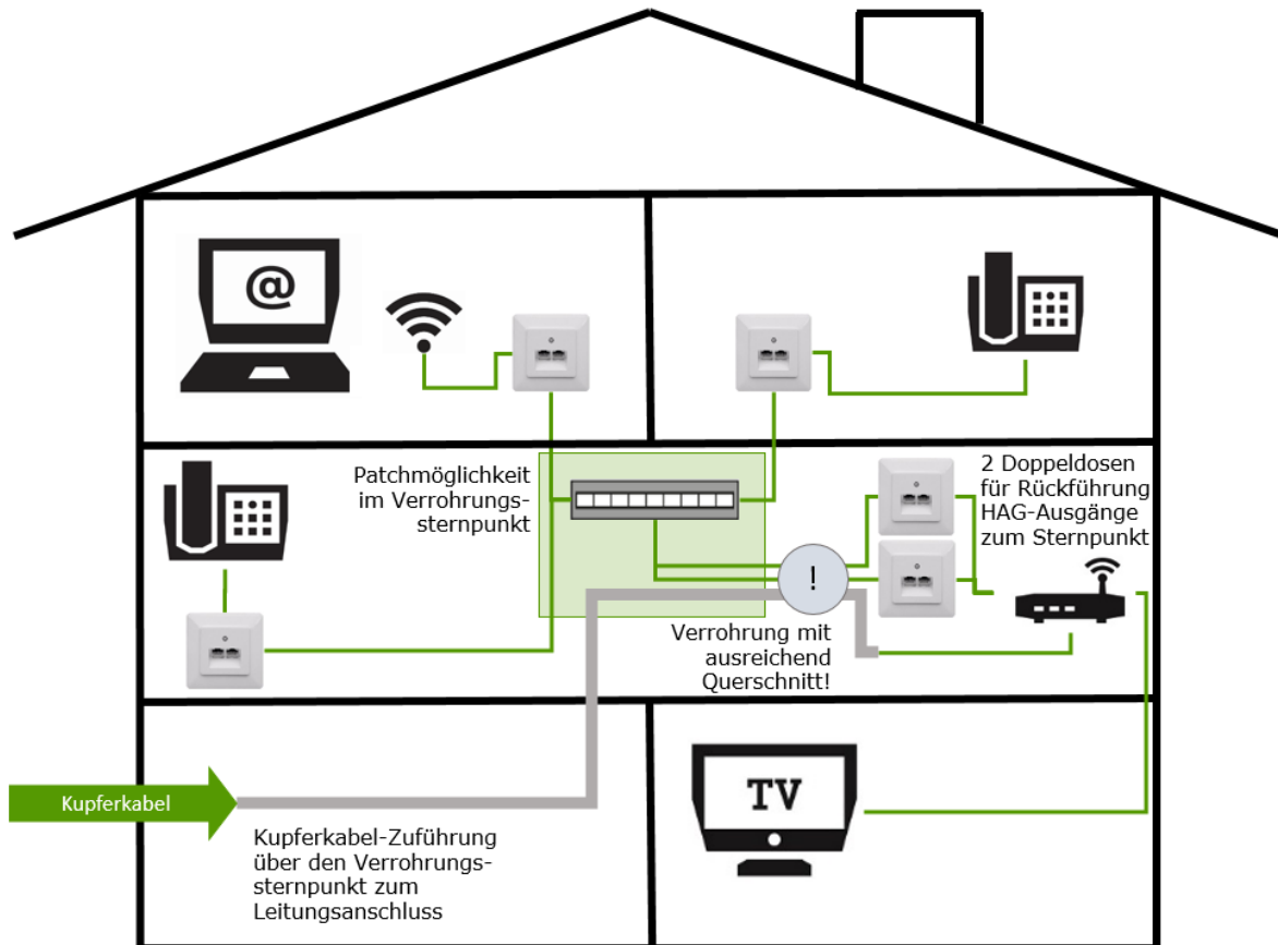
Abbildung 11: Interne Installation für Einfamilienhäuser ohne MVT
